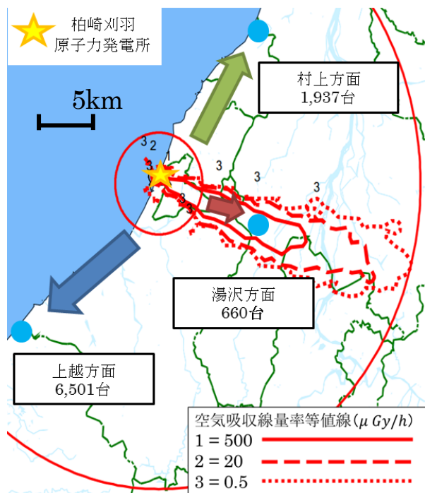
図-1 線量及び避難需要のシミュレーション条件
